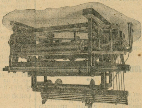
Telar F. A. 1 con 3 plegadores para Doble Tejido (Suela)
